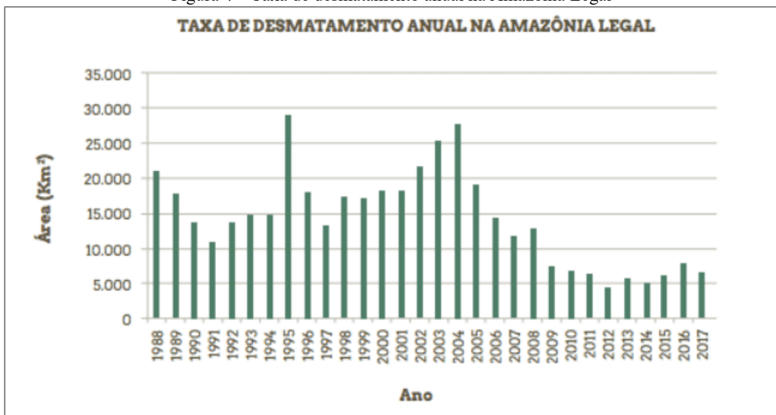
Figura 4 – Taxa de desmatamento anual na Amazônia Legal
