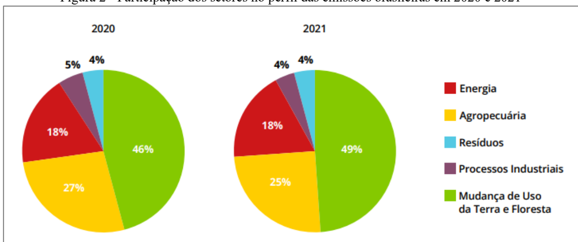
Figura 2 - Participação dos setores no perfil das emissões brasileiras em 2020 e 2021
