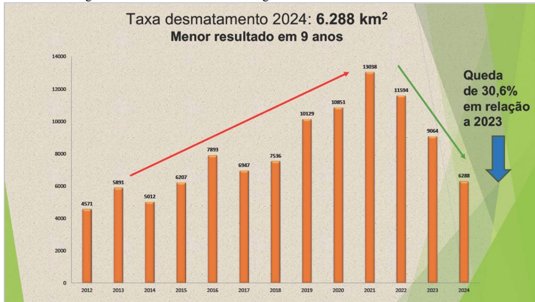
Figura 14 – PRODES Amazônia Legal 22/23: Taxa de desmatamento 2024
